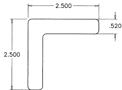
7 CORNER KEY TYPE 'B'
